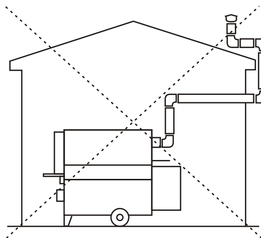
Przykłady instalacji komina odprowadzającego spaliny.
