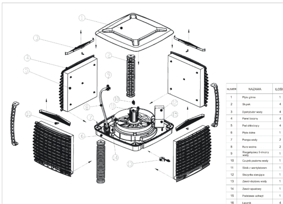
Klimatyzator Mistral 1500 (wylot dół)
