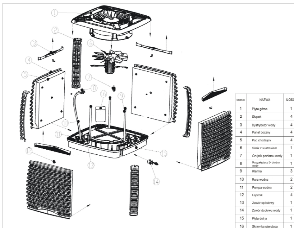
Klimatyzator Mistral 1500 (wylot góra)
